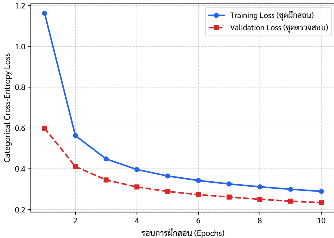
Training & Validation Loss (ฟังก์ชันสูญเสีย)
