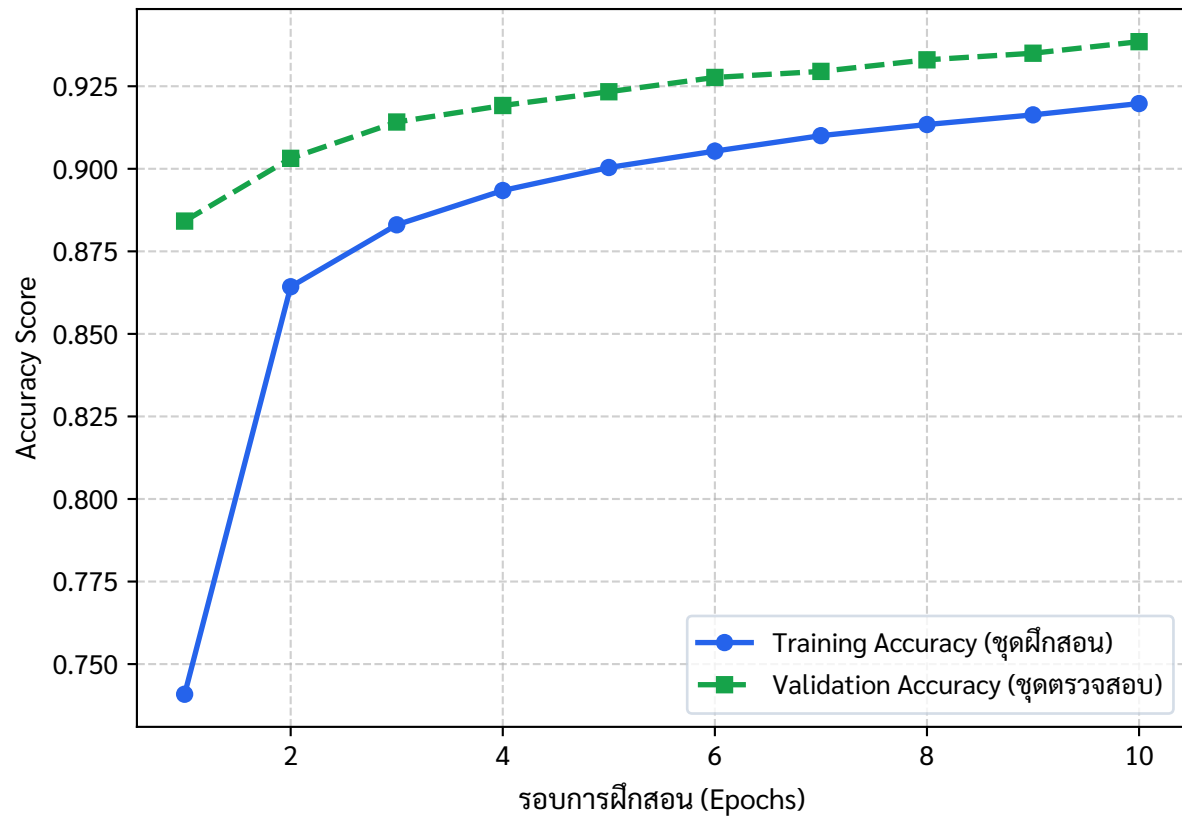
Training & Validation Accuracy (ความแม่นยำ)
